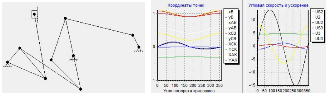
Рисунок 1 – Схема механізму переміщення основних ниток верстата типу MWWS та основна форма програми
