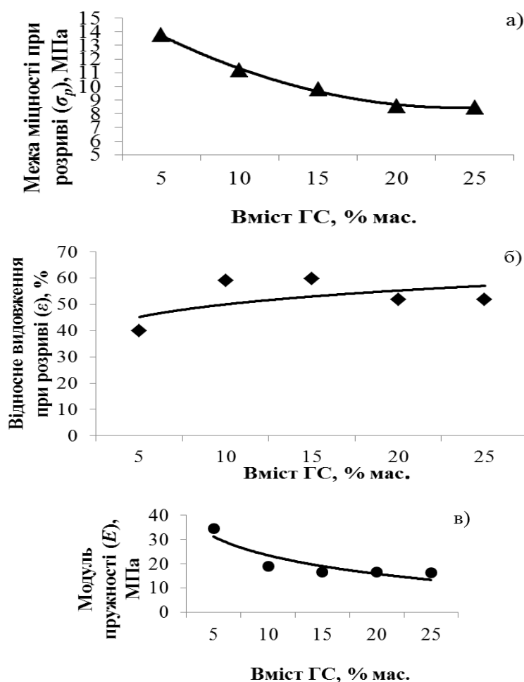
Рис. 2. Зміна властивостей ПЕ композиції від вмісту ГС:
