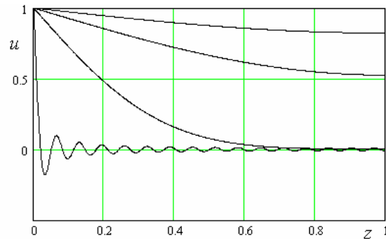
Рис.8. Динаміка зміни концентрації вологи по товщині за умови постійності коефіцієнту дифузії (вихідні дані: D = \text{const} \approx 1 \text{ c}^{-1} ; t_1 < t_2 < t_3 < t_{\text{max}} ; i = 30 )
