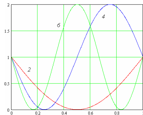
Рис.7. Графік функції f(z) = 1 - \sin\left(\frac{i \cdot \pi \cdot z}{2}\right) при i = 2, 4, 6 (парні числа)
