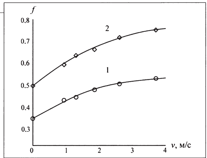
Рис. 4 – Залежність коефіцієнта тертя стрічки льону олійного вологістю 15% від швидкості ковзання: 1 – по сталі, 2 – по гумі
