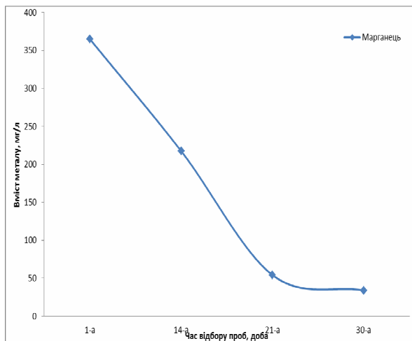
Рис. 4. Вилуговування марганцю з граншлаку силікомарганцю в амонійно-ацетатний розчин
