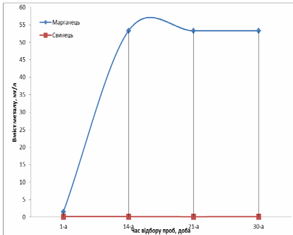
Рис. 2. Вилуговування марганцю та свинцю з граншлаку силікомарганцю у дистильовану воду
