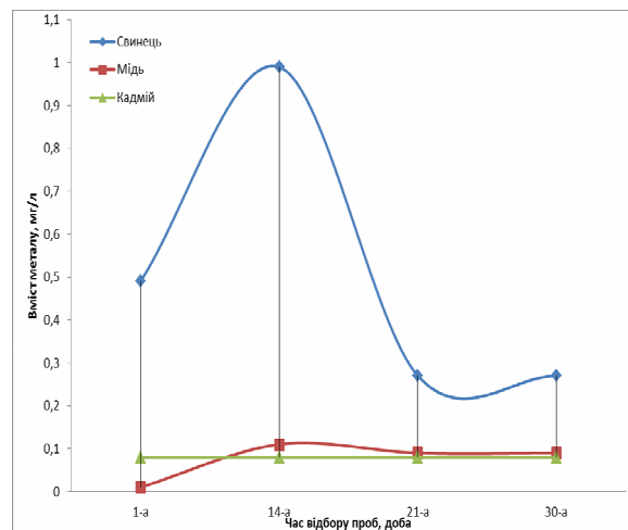
Рис. 5. Вилуговування свинцю, міді та кадмію з граншлаку силікомарганцю в амонійно-ацетатний розчин
