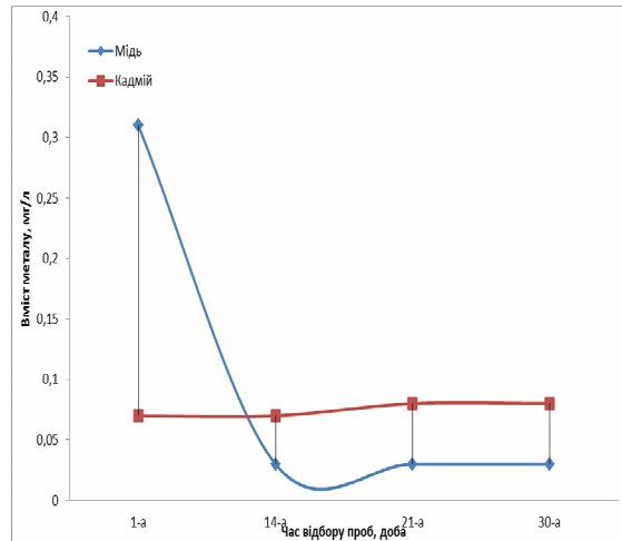
Рис. 3. Вилуговування міді та кадмію з граншлаку силікомарганцю у дистильовану воду
