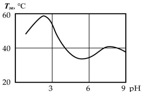
Рисуюнок 4.2 – Залежність зв'язування танідів від рН дубильної рідини
