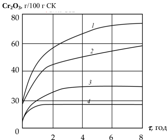
Рисунок 3.3 – Залежність кінетики зв'язування сполук хрому з голинним порошком від загальної кислотності розчину
