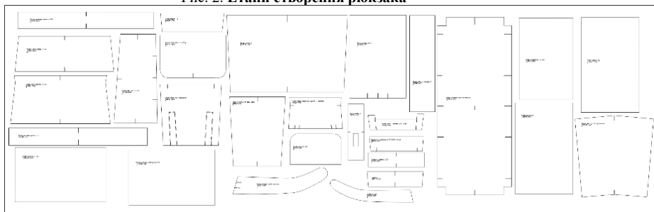
Рис. 3. Розкладка лекал рюкзака
