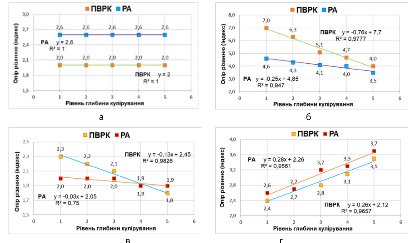
Рис. 3. Графіки залежності опору різанню (індекс) від зміни щільності в'язання: з UHMWPE нитки: а) вздовж петельного стовпчика; б) вздовж петельного ряду; з рА нитки: в) вздовж петельного стовпчика; г) вздовж петельного ряду
