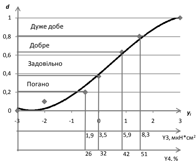
Рис. 1. Узагальнений графік функції бажаності для безрозмірного показника u_i , та показників формостійкості: жорсткості, Y_3 , та формостійкості, Y_4
