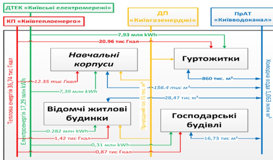
Рис. 1. Розподіл енергетичних потоків між споживачами КПШ ім. Ігоря Сікорського
