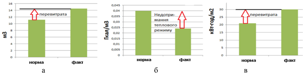
Рис. 2. Аналіз споживання енергії та води навчальним корпусом №18 а – холодна вода (на 1 особу), б – тепла енергія, в – електроенергія
