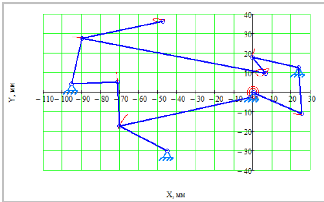
Рисунок 1 – Схема механізму зубчатої рейки швейної машини в Mathcad
